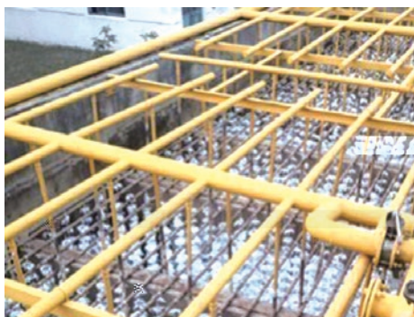
好氧池填料更換
